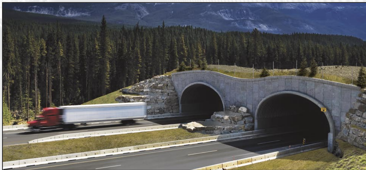
Figure 4 – Passage souterrain en tôle forte à ondulations profondes avec écrans, colliers et murs d'extrémité en béton
